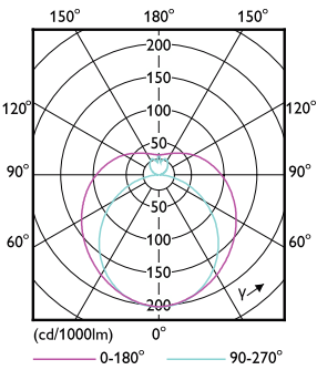
LEDtube COR 8ft 33W FA8 4400lm-LDD
