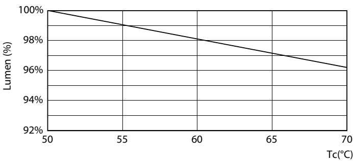
LEDtube COR 8ft 33W 50K LumenVsTc-LMP
