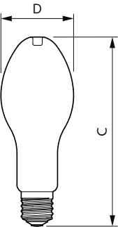
32GC/LED/850/ND E39 BB 6/1
