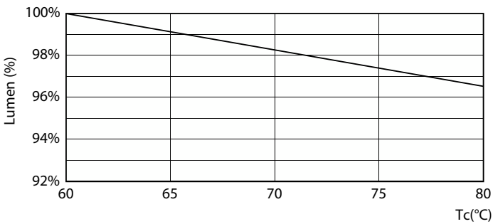
LEDtube_PLCT_8W_30K_LumenVsTc-LMP
