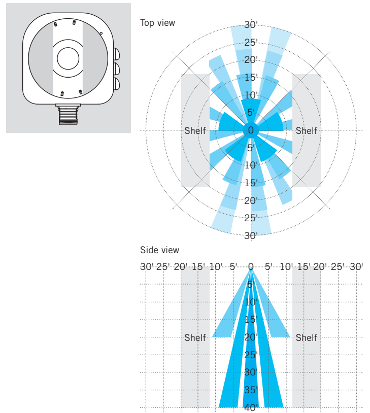
Aisle Lens
