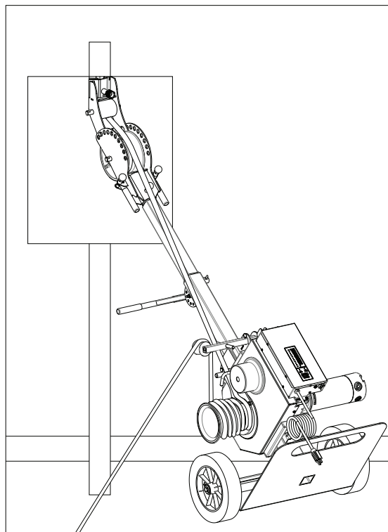
Instalación típica para una tracción descendente
