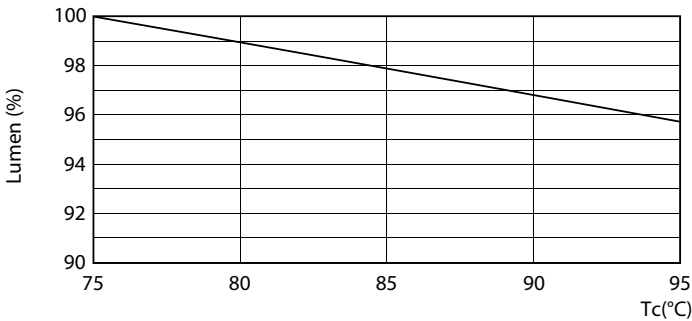
LEDtube G5 25W LumenVsTc
