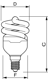
QSPIR-F 23W/827 E26 110-127V Spiral
