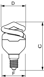
QSPIR-F 23W/827 E26 110-127V Spiral
