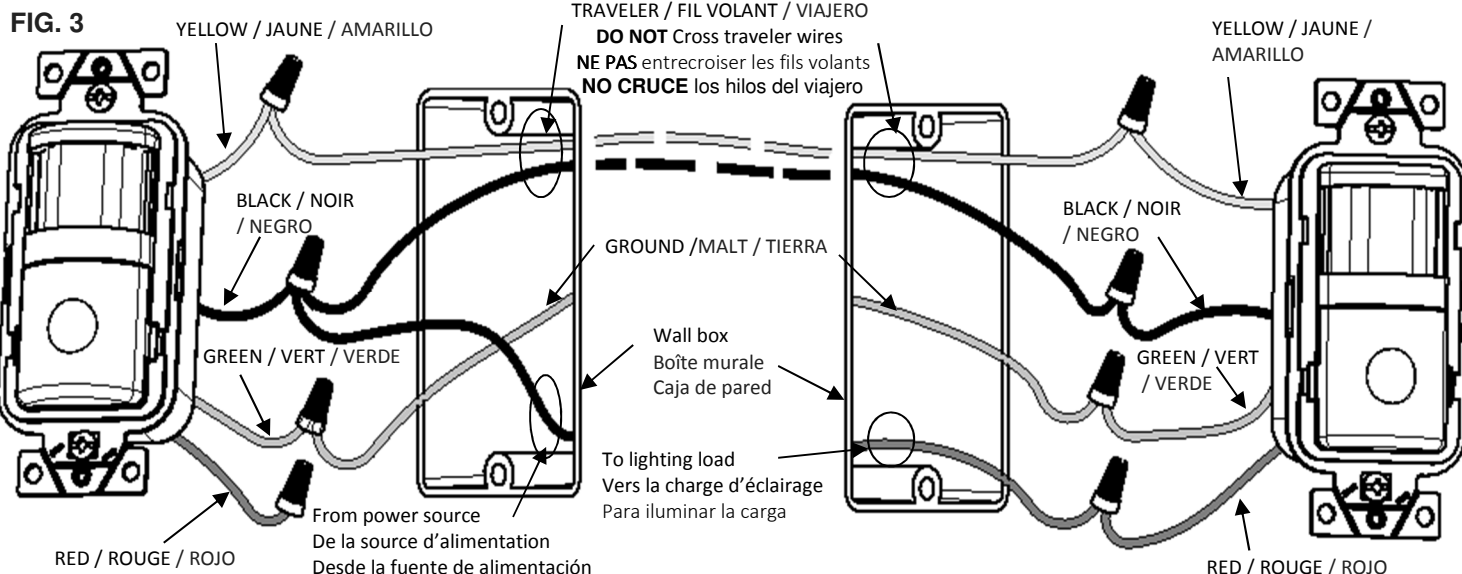
3-Way Wiring / Câblage 3 voies / Cableado 3 modos
