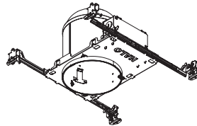
HALO® Housing (Sold separately) Boîtier HALO® (vendu séparément) Alojamiento HALO® (vendido por separado)
