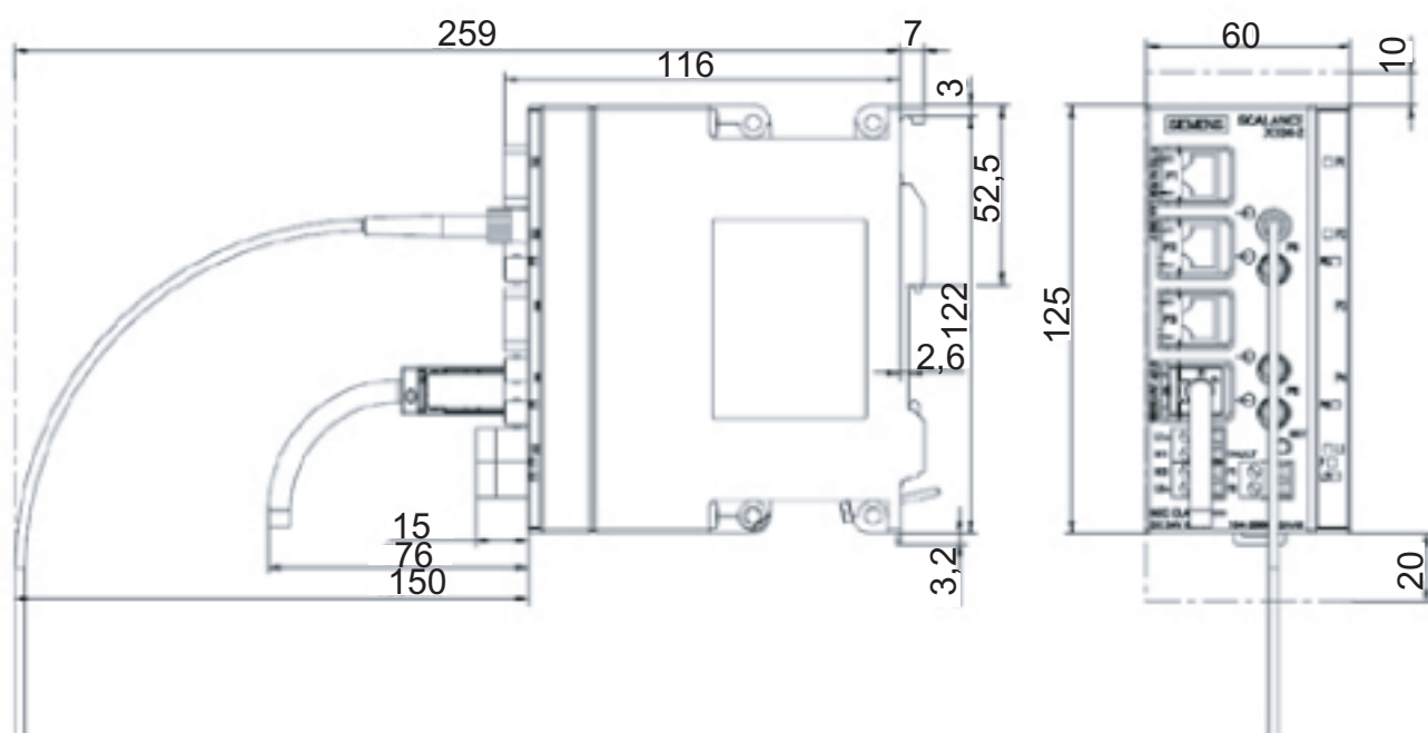
Bild 8-4 SCALANCE X200 Seitenansicht
