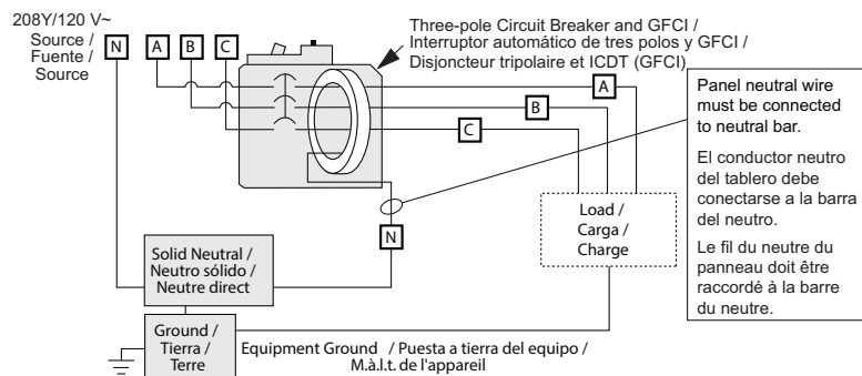
FIG. 3 : Multi-Wire Circuits / Circuitos de múltiples hilos / Circuits multifilaires
