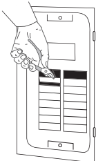
FIG. 2 : Removing Twist-Out / Desmontaje de los rectángulos removibles / Retrait des plaquettes à tordre
