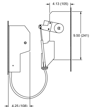
9422CSJ 3-Pole
