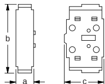
Main Pole Module
