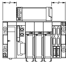
Racks TSX RKY 6 / 6E
