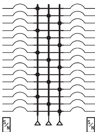
125–250 A Main Lugs
