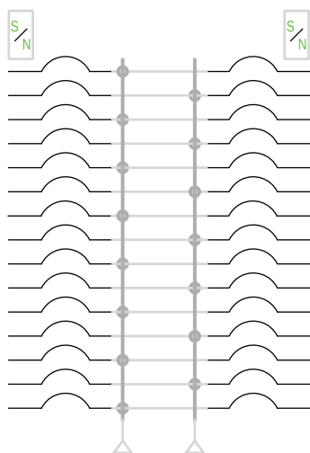
NF 800 A Main Lugs
