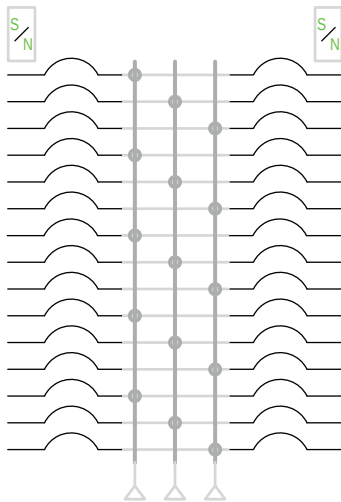
NF 800 A MLO—3PH, 4W
