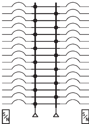
125–250 A Main Lugs
