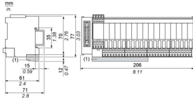
(1) ABE7BV20 / ABE7BV20E
