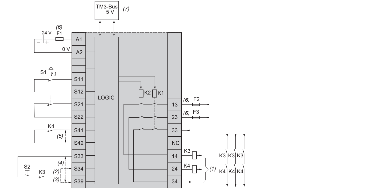
Wiring diagram / Schéma de câblage / Anschlussbild / Diagrama de cableado / Schema di cablaggio / 接线图
