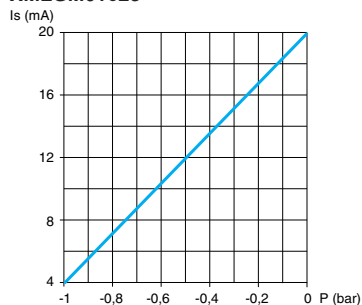
XMLGM01●23
