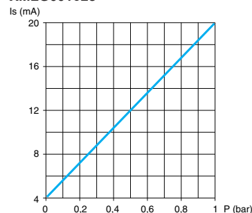
XMLG001●23
