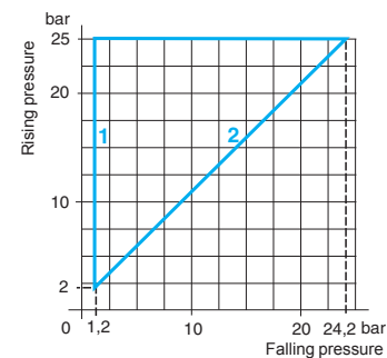
XMLG025●●1
