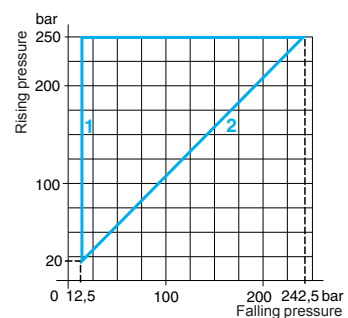
XMLG250●●1TQ
