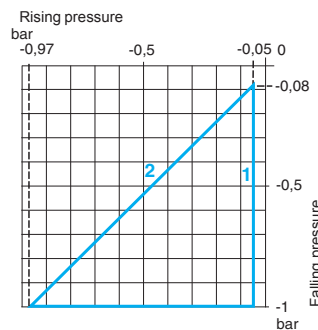
XMLGM01●●1
