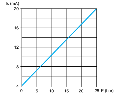
XMLG025●23
