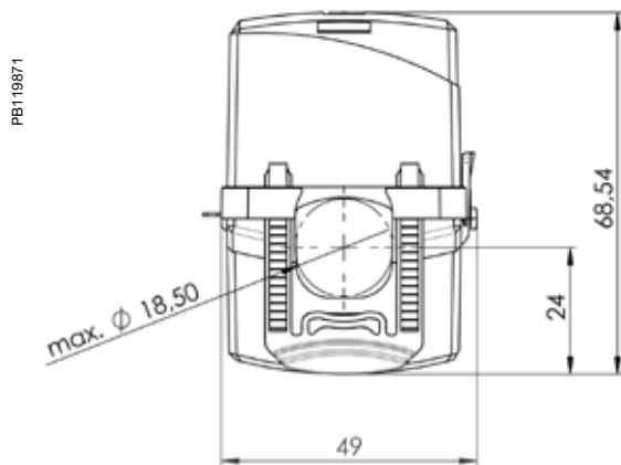
HA Dimensions
