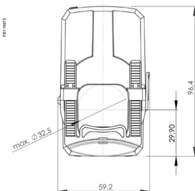
HG Dimensions
