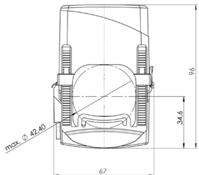
HJ Dimensions
