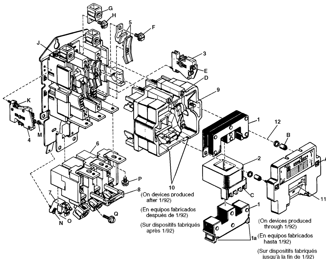
Figure / Figura / Figure 1 : Contactor and Starter Assembly / Ensemble de contacteurs y arrancadores Assemblage de contacteur et de démarreur
