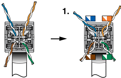
Cable End 2
