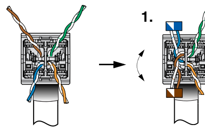
Cable End 2
