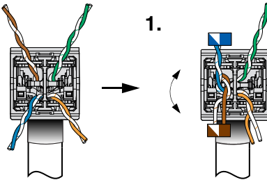
Cable End 2
