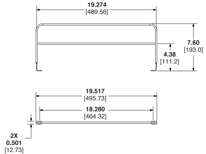
SRB19D7BL
