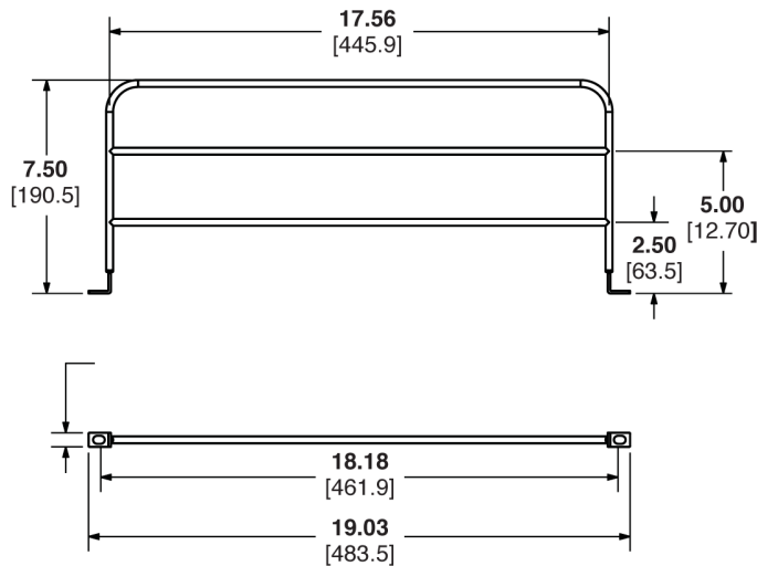
SRB19MDBL
