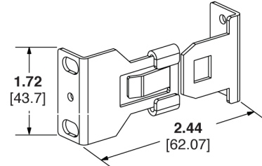
SRBBRKT
