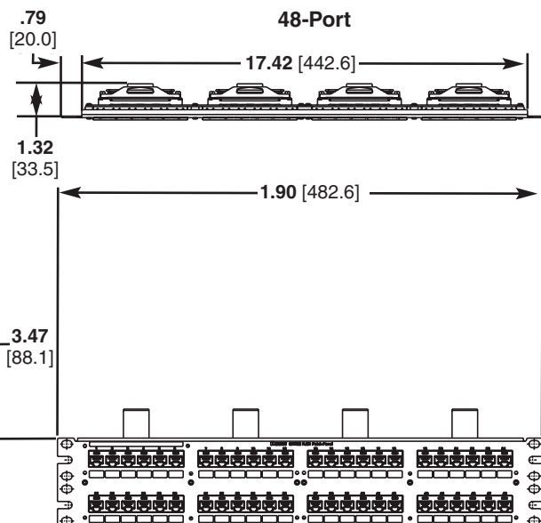
48-Port
