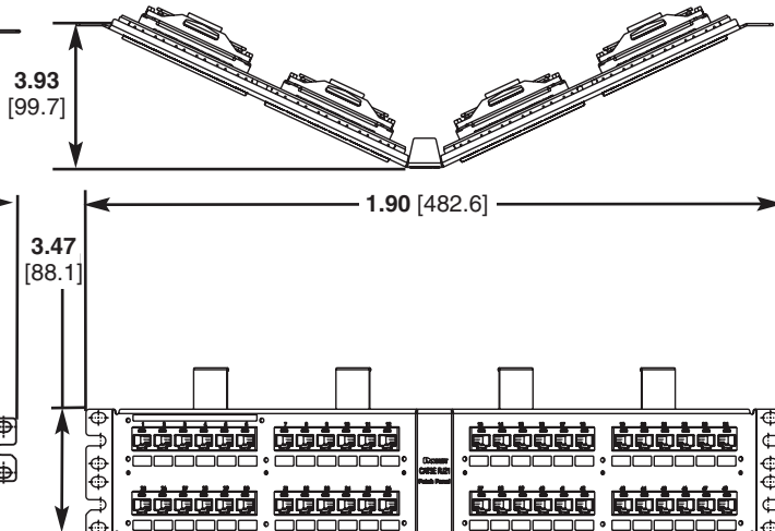
48-Port Angled
