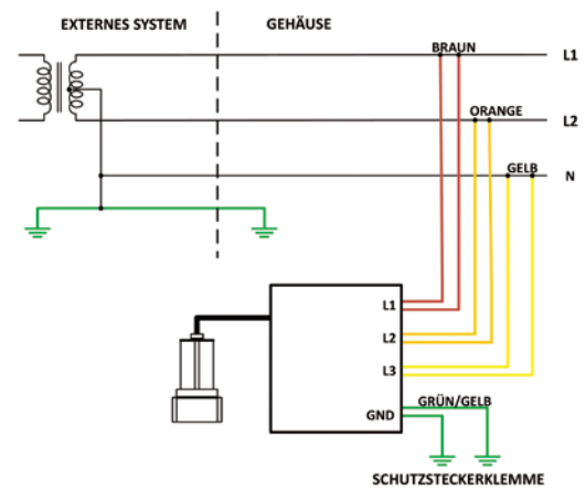
Einphasen: Dreiadrig + PE
