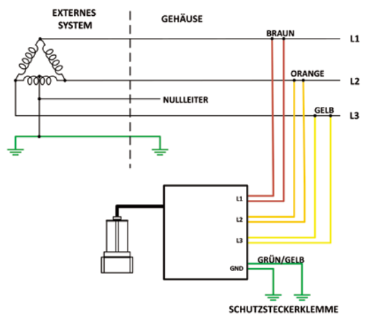
High-Leg-Delta: Dreiadrig + PE
