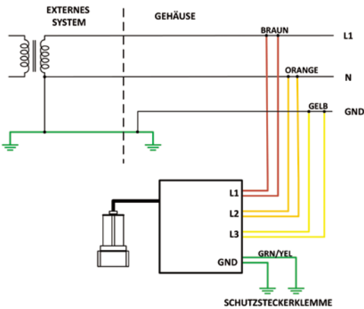
Einphasen: Zweiadrig + PE
