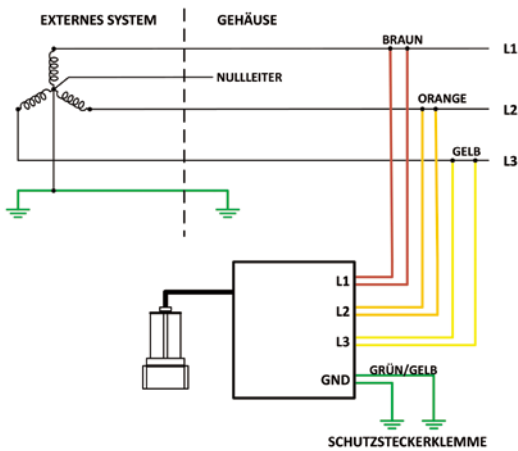
Dreiphasen-WYE: Dreiadrig + PE (kein Nullleiter)
