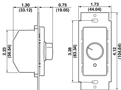
Sélecteur de lampe/bouton de programmation
