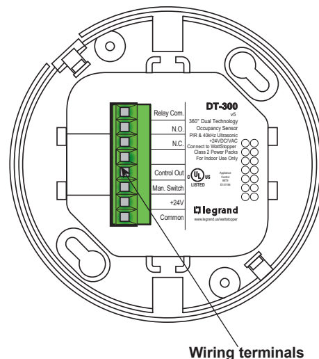
Wiring terminals
