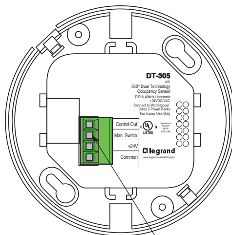
Wiring terminals
