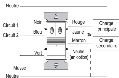
Câblage à double circuit des PW-302-347
