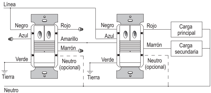
Cableado de dos niveles (PW-302-347 – hasta 4 sensores)
