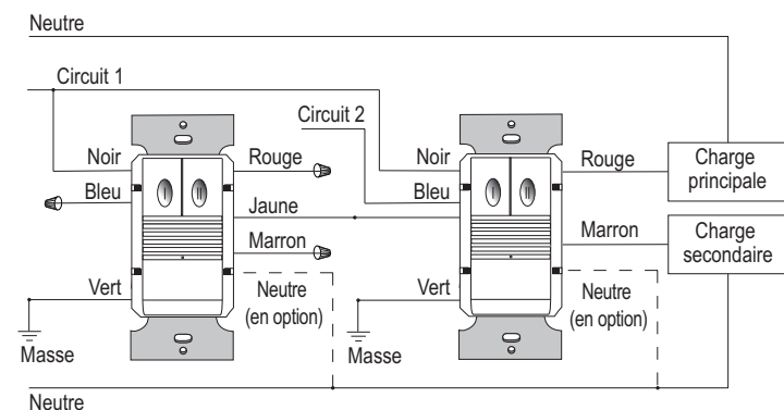
Câblage biphase
