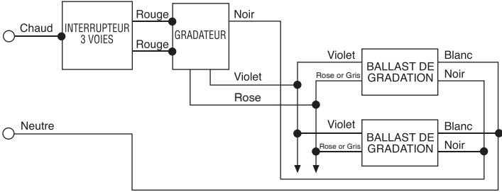
Figure 2 – câblage 3 voies
