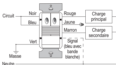
Câblage à deux niveaux des PW-302
