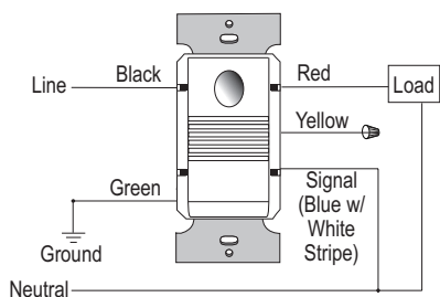
PW-301 Wiring
