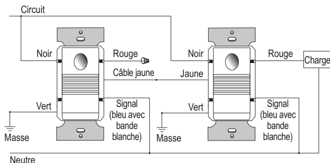
Câblage standard (PW-301 - jusqu'à 4 détecteurs)
