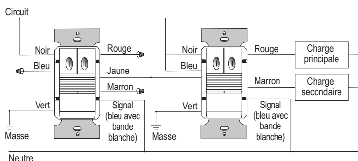
Câblage à deux niveaux (PW-302 - jusqu'à 4 détecteurs)
