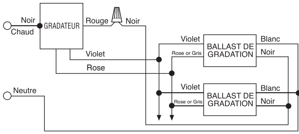
Figure 2 – câblage 3 voies
