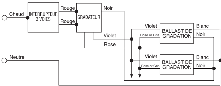
Figure 2 – câblage 3 voies
