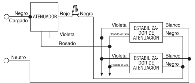
Figure 2 – Cableado de 3 vías
