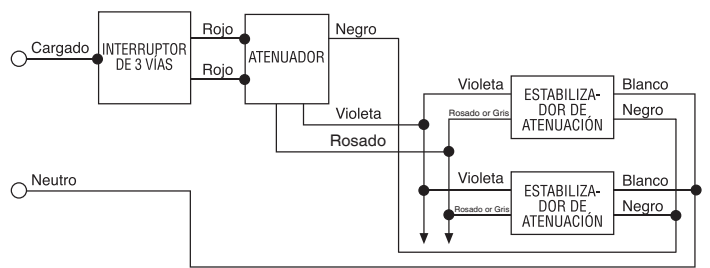
Figure 2 – Cableado de 3 vías
