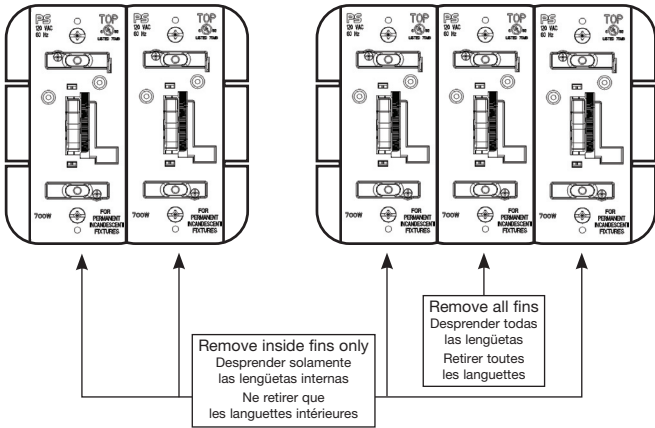
Figure 2: Multiple Ganging of devices Figura 2: Instalación en grupo de múltiples dispositivos Figure 2 : Groupement de plusieurs dispositifs
