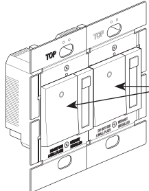
2-Gang Installation Installation 2 variateurs Instalación de 2 juegos Remove inside fins only Retirer les plaques situées à l'intérieur uniquement Retire solo las aletas internas
