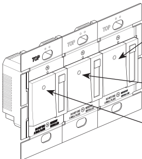
3-Gang Installation Installation 3 variateurs Instalación de 3 juegos Remove inside fins only Retirer les plaques situées à l'intérieur uniquement Retire solo las aletas internas Remove all fins Retirer toutes les plaques Retire todas las aletas Remove inside fins only Retirer les plaques situées à l'intérieur uniquement Retire solo las aletas internas
