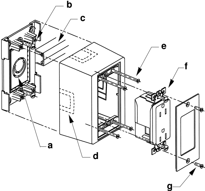
Fig. 4 Single Gang Device Box / Boîte de dispositif simple / Caja de dispositivo simple PW1LPB, PW1SBA, PW1DBA
