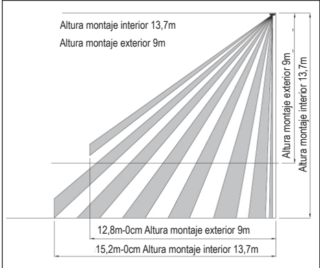
Fig. 7 - Vista lateral del rango de cobertura de la lente a 9 y 13,7m (30 ft & 45 ft)
