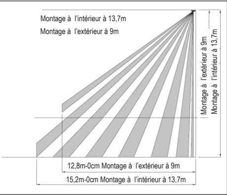
Fig. 7 – Vue latérale de la portée à 9 m et 13,7 m
