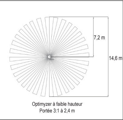
Fig. 6 – Vue en plongée de la portée de la lentille à 2,4 m
