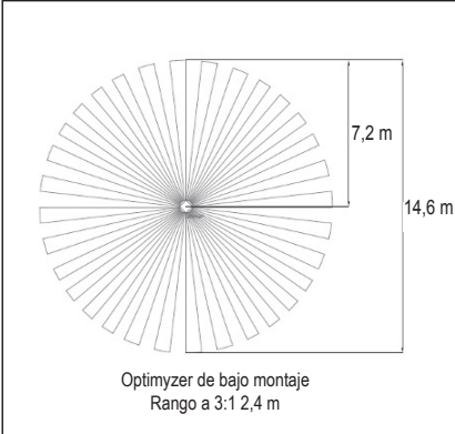
Fig. 6 – Vista superior del rango de cobertura a 2.4 m (8 ft)
