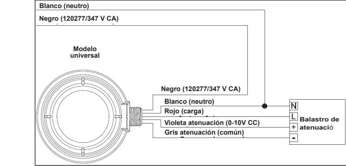
Fig. 3 - Diagrama eléctrico A - 120/277/347 V CA diagrama eléctrico de tensión de línea
