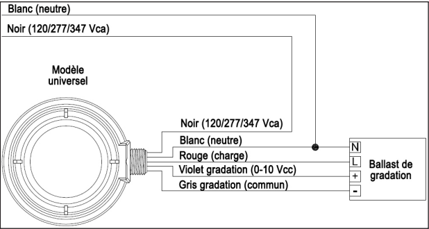
Fig. 3 - Schéma de câblage A – tension de ligne 120/277/347 Vca
