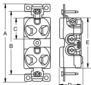
Duplex Receptacle
