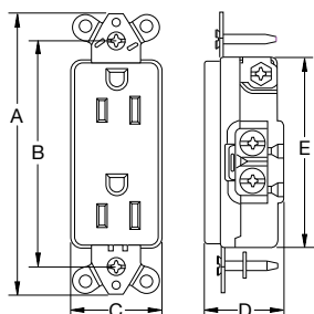
Duplex Receptacle
