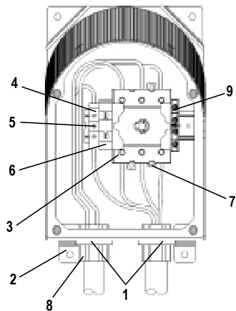
Fig. M-2
