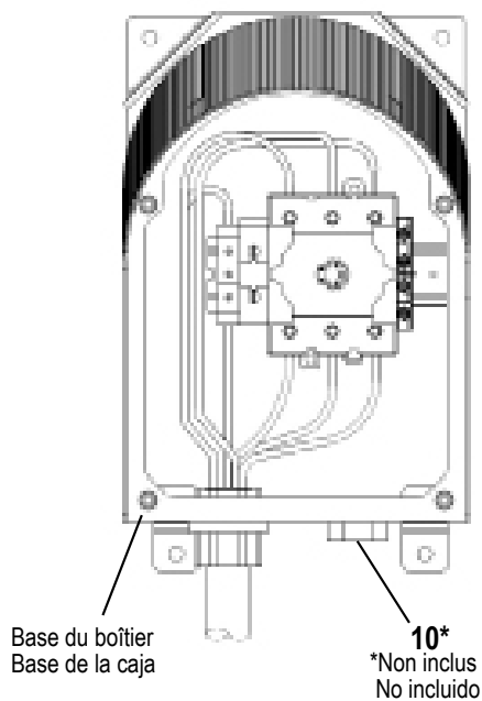
Fig. M-3
