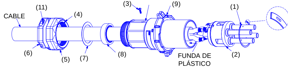
FIGURA 1 • CLAVIJA
