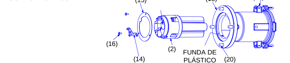
FIGURA 3 • TOMACORRIENTE
