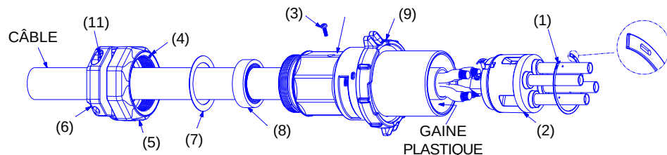
FIGURE 2 • CONNECTEUR
