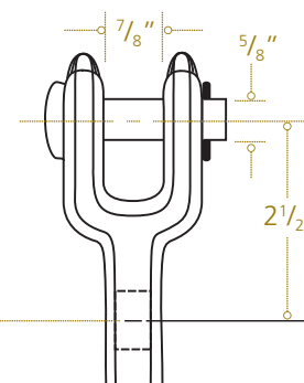
Clevis Type CA
