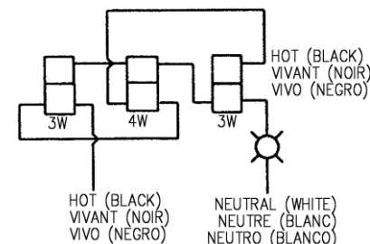
4 Way 4 Voies 4 Vías
