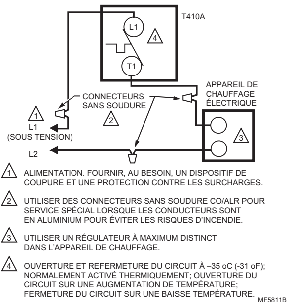
Fig. 2. Raccordement type d'un T410A.
