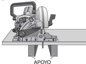
FIG. 15 NO apoye la tabla o el panel LEJOS del corte.
