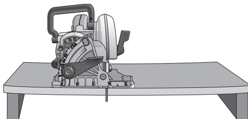
FIG. 15 NO apoye la tabla o el panel LEJOS del corte.
