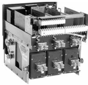
DSII308—Rear
