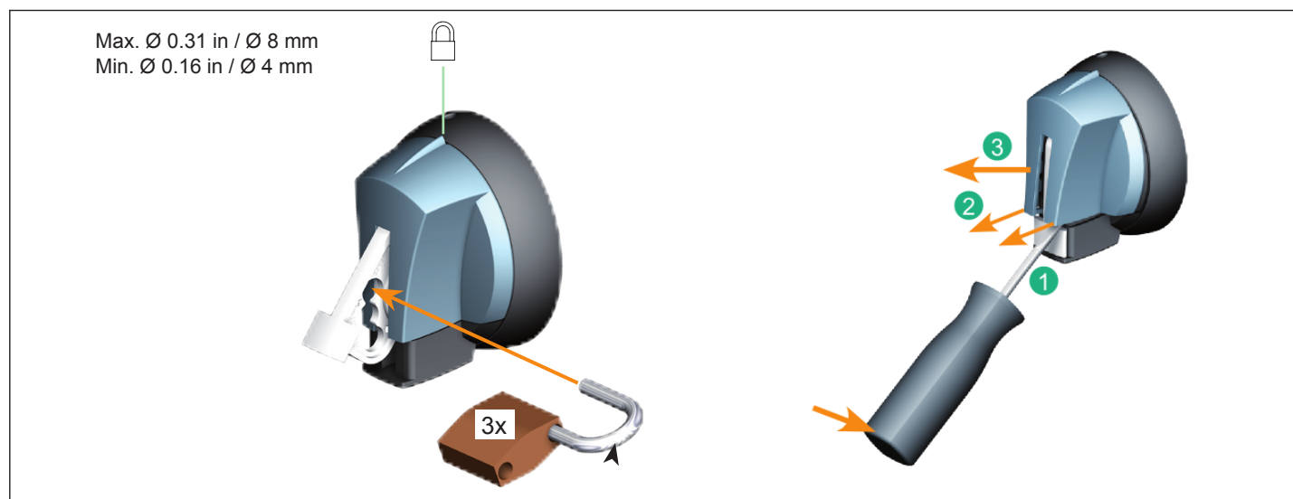
Figure 3. Padlocking the Handle / Cadenassage de la Poignée / Bloqueable Para Candados
