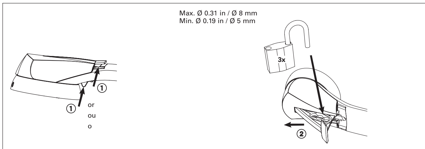
Figure 3. Padlocking the Handle / Cadenassag de la Poignée / Bloqueable Para Candados
