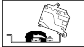
Figure 4. Step 7—Install CH Branch Circuit Breakers / Figura 4. Paso 7 - Instalación de interruptores de circuito de derivación tipo CH
