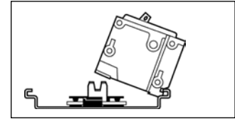
Figure 5. Step 7—Install BR Branch Circuit Breakers / Figura 5. Paso 7 - Instalación de interruptores de circuito de derivación tipo BR
