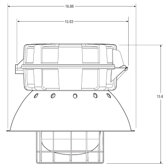
Pendant mount
