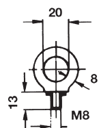
Eyebolt A2
