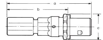
Fig. 7 - NPJ Plugs
