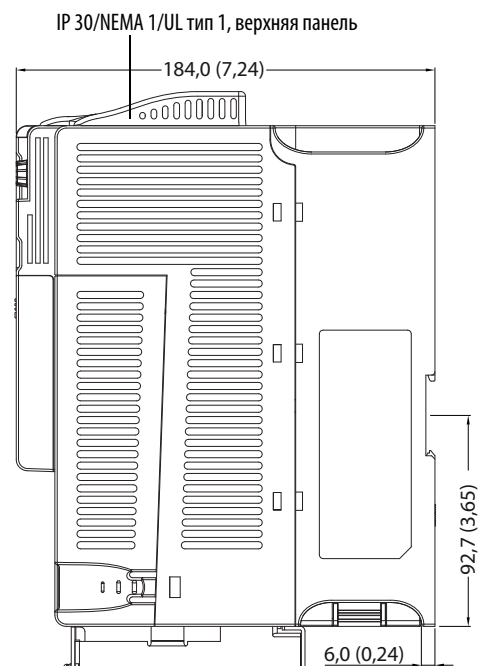
IP 30/NEMA 1/UL тип 1, распределительная коробка
