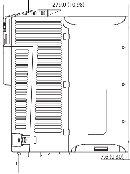
IP 30/NEMA 1/UL тип 1, распределительная коробка
