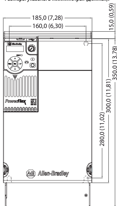
IP 30/NEMA 1/UL тип 1, верхняя панель
