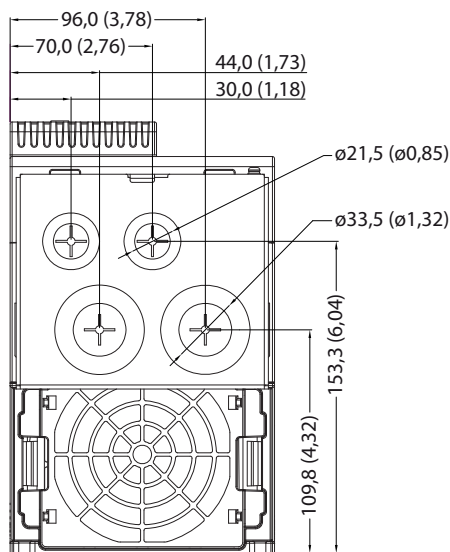
IP 30/NEMA 1/UL тип 1, распределительная коробка
