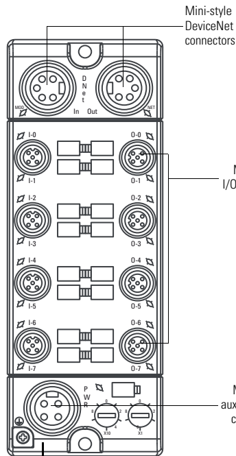
16 Point I/O Modules
